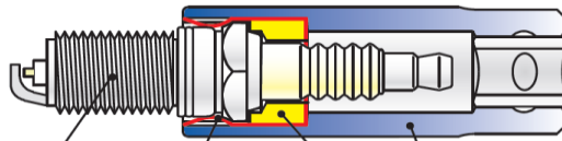
Bougie Ressort de maintien Laiton Corps de douille
